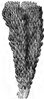
Fig. 69.— Azorella selago .
